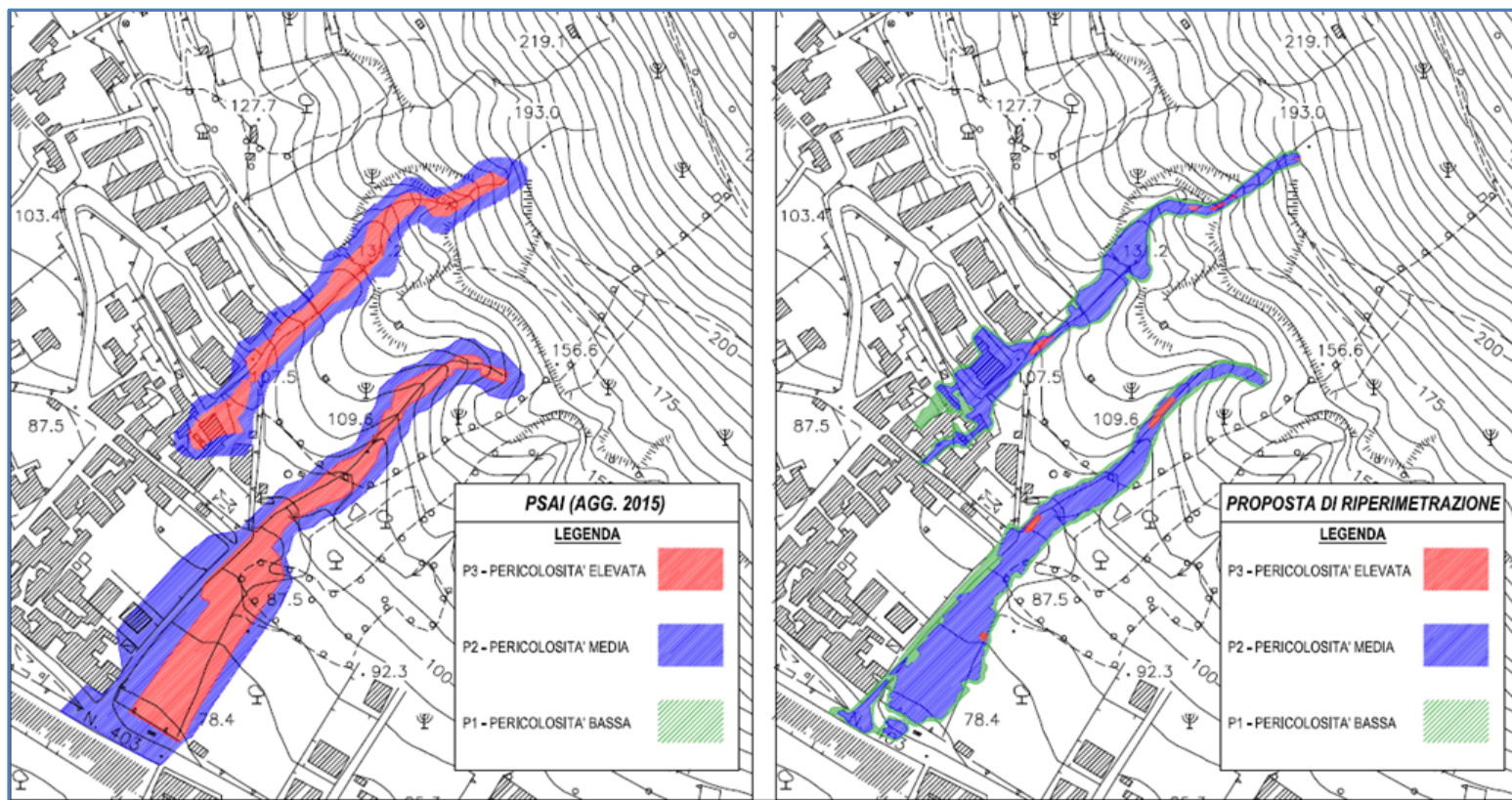
Comune di Liveri (NA)– via Salita Stella,- Piano Stralcio di Assetto idrogeologico dell'ex AdB Campania Centrale - Stralcio mappa della pericolosità idraulica vigente (sx) Stralcio mappa della pericolosità idraulica proposta (dx) -tav. 448072P.
